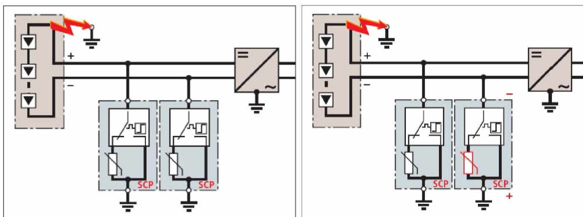
Фиг.9.18.1.3 Пробив в изолацията на PV генератор Фиг.9.18.1.4 Претоварване на SPD, причинено от пробив в изолацията
